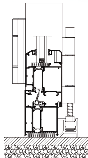
Detalle guía superpuesta
