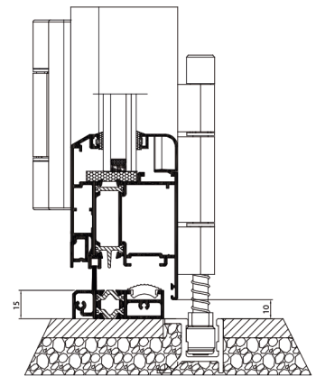
Detalle guía encastrada con umbral
