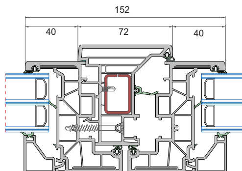
Sección horizontal
