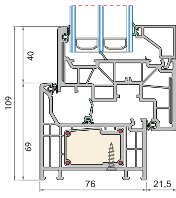
Sección vertical
